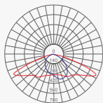
SL-1A 150°x70°
