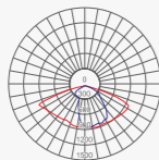
SL-2A 150°x70°
